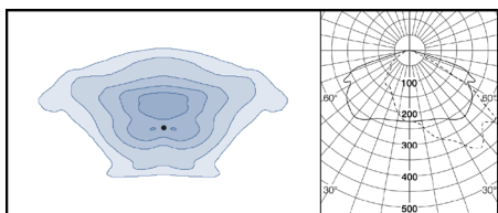
L7 Optik för stadsnära motorvägar, bostadsgator.
