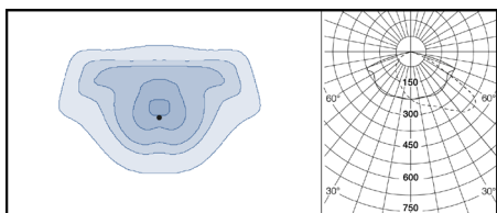
L2 Optik för stadsnära motorvägar, bostadsgator.
