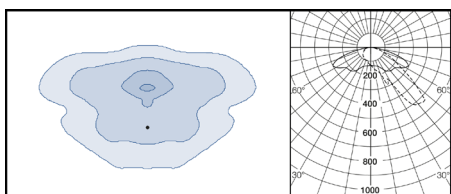
L5 Optik optimerad för god jämnhet. Stadsnära motorvägar, bostadsgator. Klarar längre stolpavstånd än L4.
